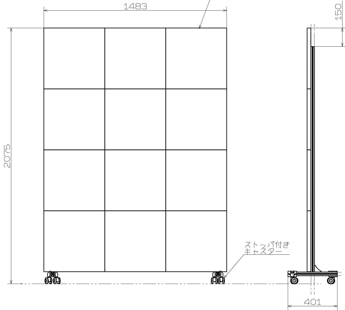
右側面図 (1:15)
